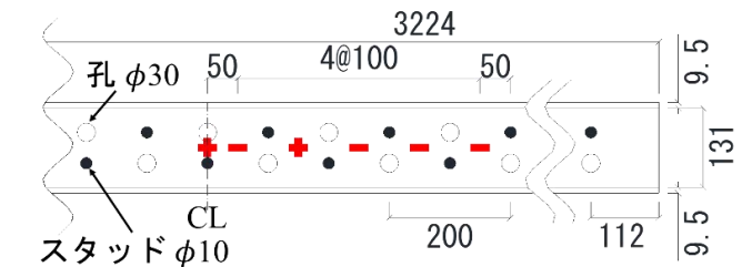
図-3 ウェブ詳細図
