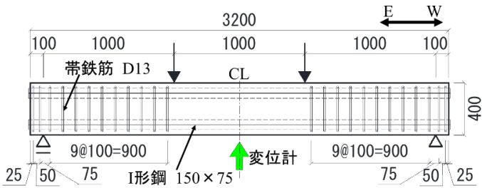
図-2 側面図
