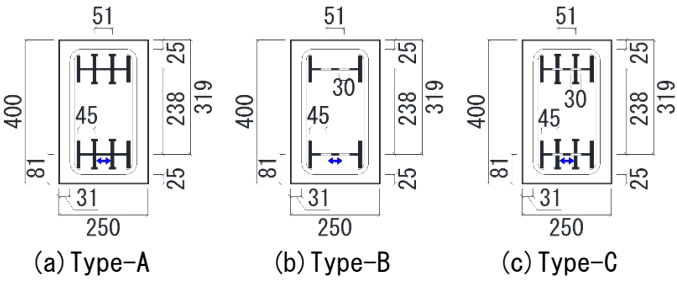
図-1 断面図
