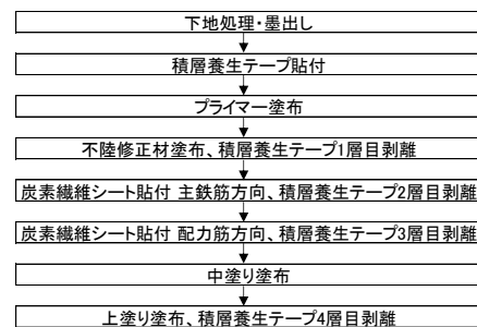
図-2 施工の流れ
