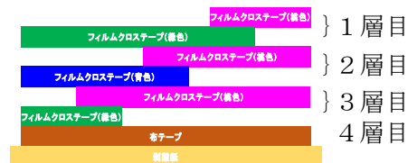
図-1 積層養生テープ 断面図
