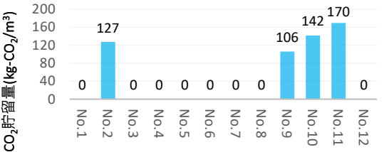
図-3 地盤改良施工による CaCO 3 としての CO 2 貯留量
