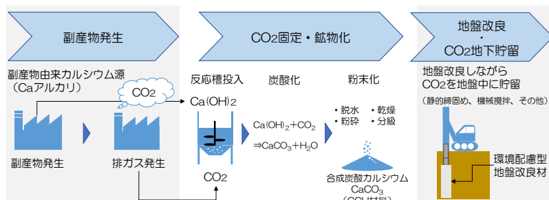
図-1 地盤改良をしながら CO 2 を地盤中に貯留する技術の模式図
