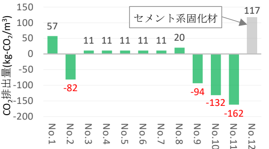
図-3 地盤改良材の CO 2 排出量
