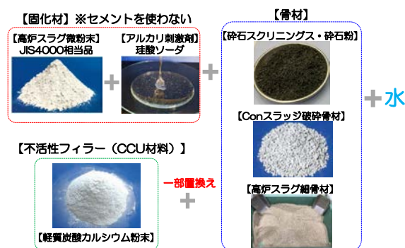
図-2 環境配慮型地盤改良材の組成
