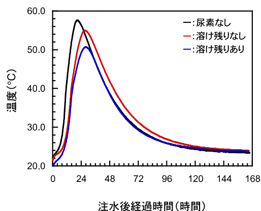
図2 簡易断熱温度上昇試験の結果
