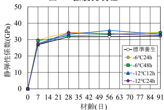
図-4 ヤング率の発現性
