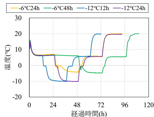
図-2 供試体内部温度計測結果
