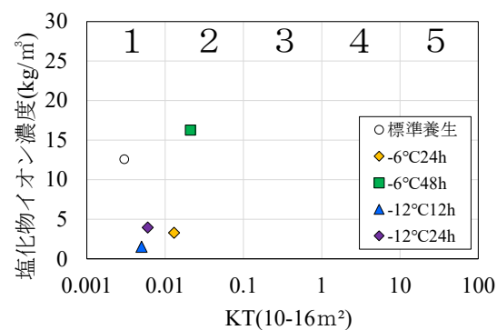
図-5 透気係数と表層部塩化物イオン濃度の関係
