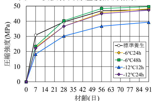
図-3 強度発現性
