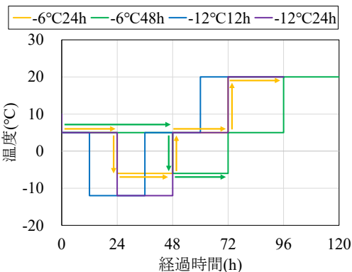
図-1 実験温度プログラム
