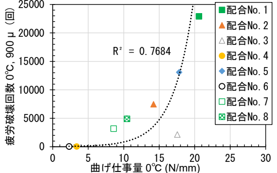
図-3 疲労破壊回数（0℃，900μ）と曲げ仕事量（0℃）の関係
