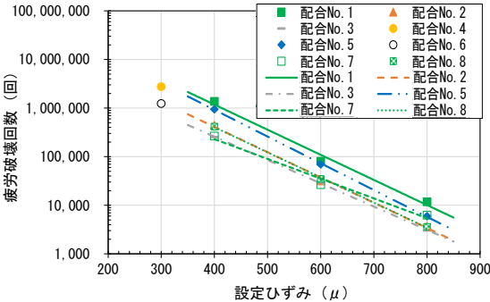
図-2 0℃曲げ疲労試験結果
