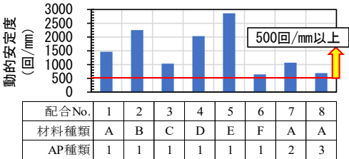
図-1 ホイールトラッキング試験結果
