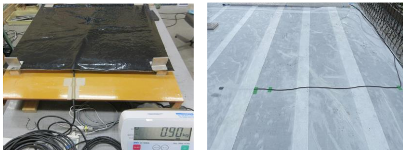
写真.1 養生マット含水率の測定 (左：室内実験、右：現場実験)
