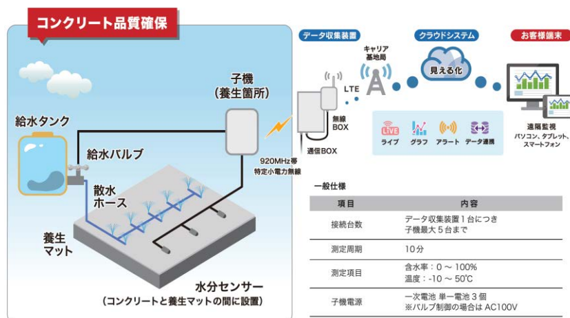
図.1 養生の自動管理システム
