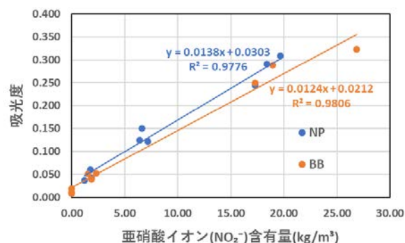
図-2 吸光度と亜硝酸イオン濃度の関係 (モルタル, 塗布後 1 ヶ年, セメントの種類)
