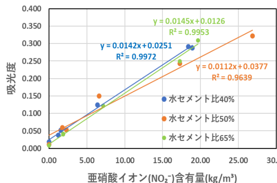
図-3 吸光度と亜硝酸イオン濃度の関係 (モルタル, 塗布後 1 ヶ年, 水セメント比)
