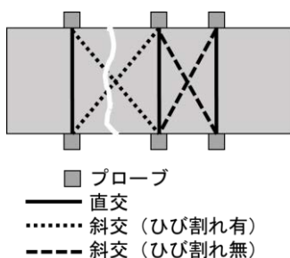
図-2 直交・斜交法
