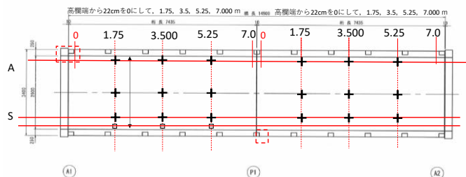
図-4 ハンマー打撃とセンサーの位置
