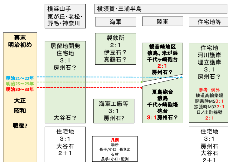
図-2 ブラフ積み石垣整備様式の変遷
