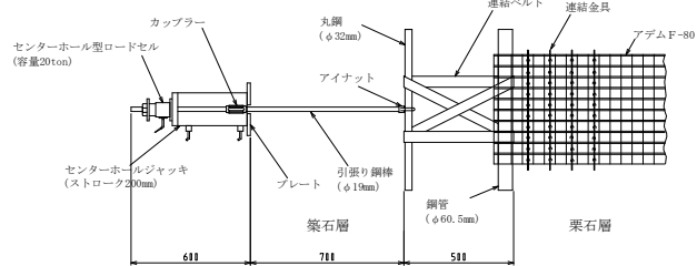
図-4 引抜き試験の概要図
