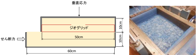
図-1 一面せん断試験模式図 写真-2 ジオグリッド設置状況
