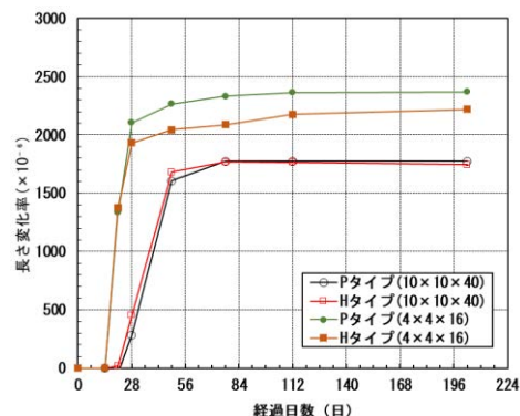
図-2 経過日数に対する体積変化
