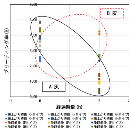
図-3 経過時間に対するブリーディング率
