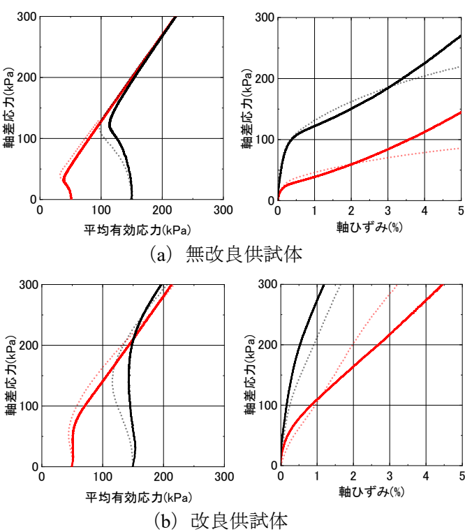
図 2 Dr=40%の試験結果及び計算結果 (実線：試験結果, 点線：計算結果)
