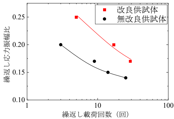
図 1 液状化強度曲線 (Dr=40%)
