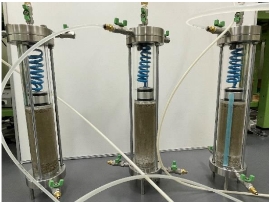
写真 1 養生中の三軸供試体
