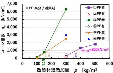
図 2 配合試験結果
