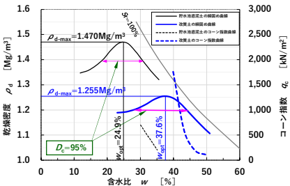
図-3 改質土の締固め曲線
