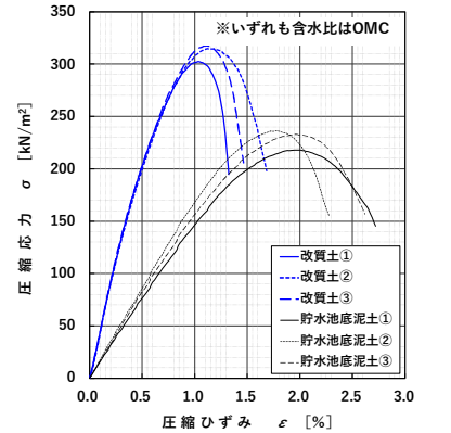
図-5 改質土の応力~ひずみ曲線
