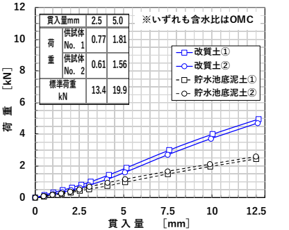
図-4 改質土の荷重~貫入量曲線
