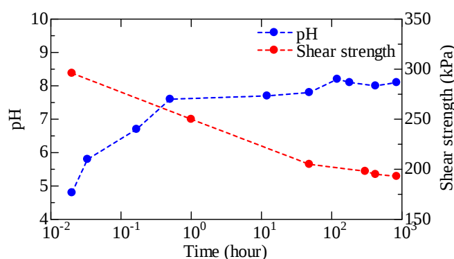
図4 浸漬時間とpH・非排水せん断強度の関係
