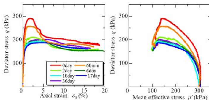
図2 溶脱時間の違いによる非排水せん断挙動
