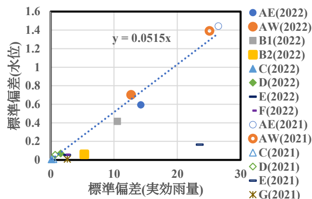
図-5 実効雨量・水位の標準偏差
