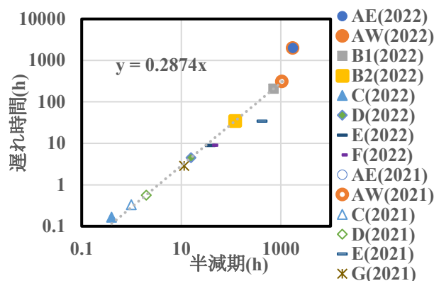
図-3 半減期と遅れ時間
