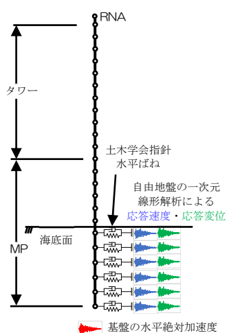
図2 解析モデル
