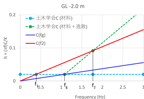
図4 GL-2mの減衰定数
