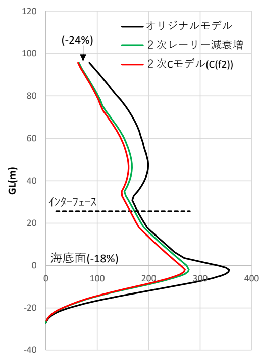
図6 曲げモーメント応答の比較 (MNm)
