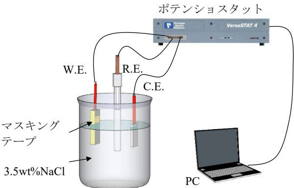
図-2 電気化学測定の模式図
