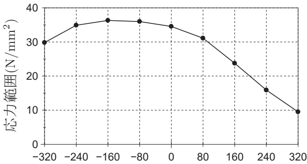
図-6 着目点の応力範囲
