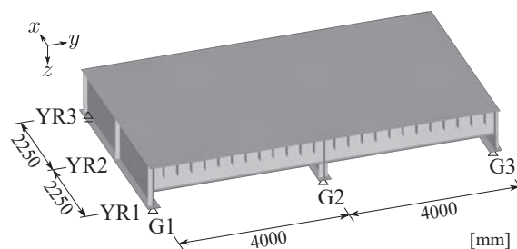
図-2 解析モデル全体図
