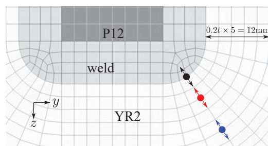
図-3 P12とYR2との交差部近傍の着目点
