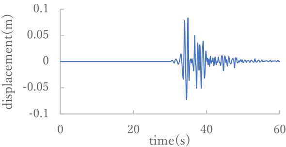
図 4 兵庫県南部地震、変位
