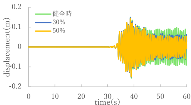
図5 主桁スパン中央の応答変位
