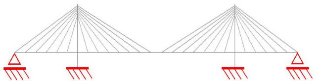
図 3 解析モデルの境界条件
