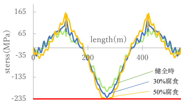
図6 主桁最大圧縮応力
