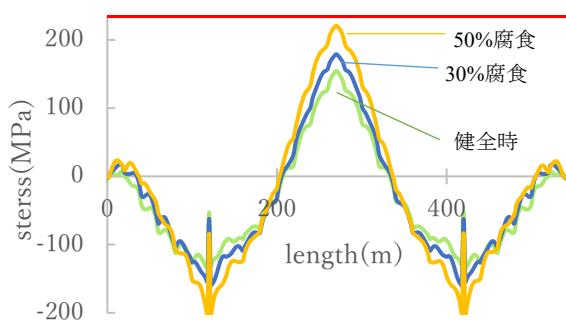
図7 主桁最大引張応力
