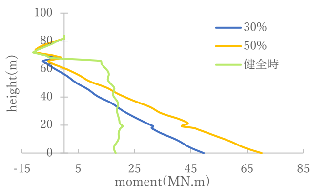
図8 主塔基部の曲げモーメント分布
