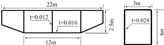
図 2 主桁、主塔断面
