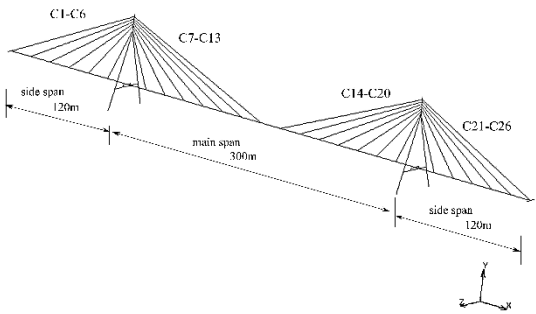
図 1 斜張橋モデル
