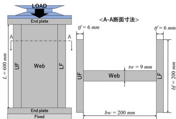
図-1 試験体の概形
