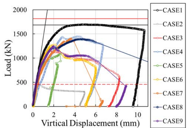
図-2 荷重－鉛直変位関係
