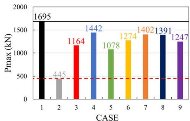
図-3 最大荷重
