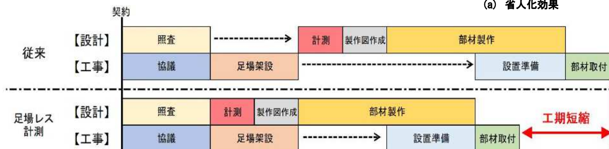
(b) 工程の比較 図-5 工程の短縮化
