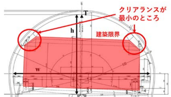
図1 道路トンネルの建築限界
