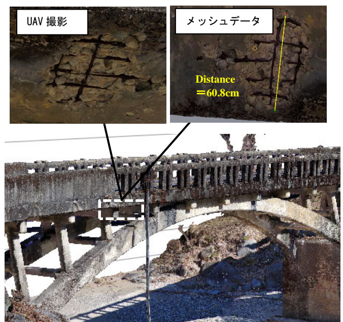
図-3 構造物全体の3Dモデル化例
