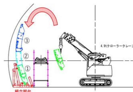
図-4 側フォーム組立検討
