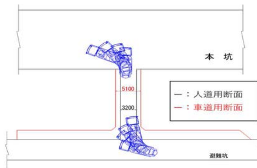
図-2 10t アジテーター車軌跡検討図
