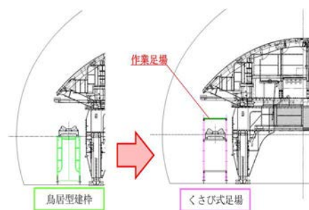
図-3 くさび式足場
