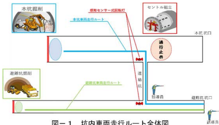
図-1 坑内車両走行ルート全体図
