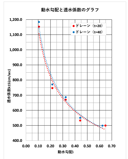
図6 動水勾配と透水係数のグラフ
