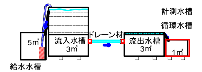
図4 透水試験水槽側面図
