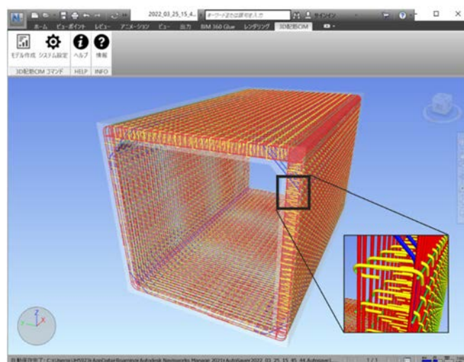
図-4 自動生成配筋モデル
