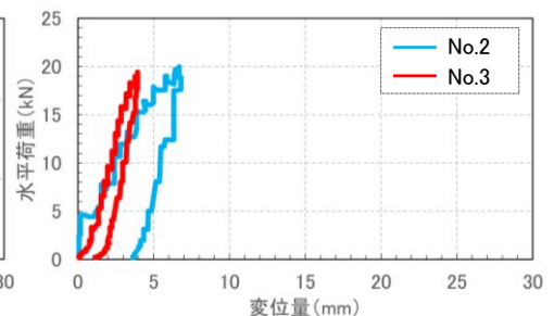
図-11 水平載荷試験結果(100 mm)
