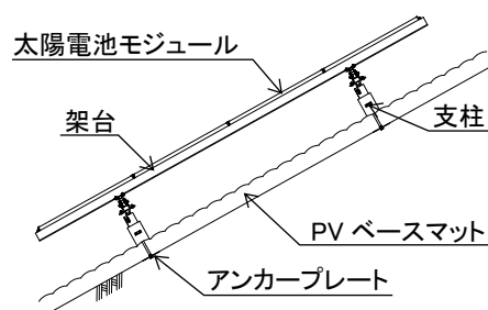
図-1 PV ベースマット工法概要図
