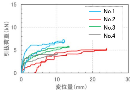
図-7 引張荷重と変位量(50 mm)
