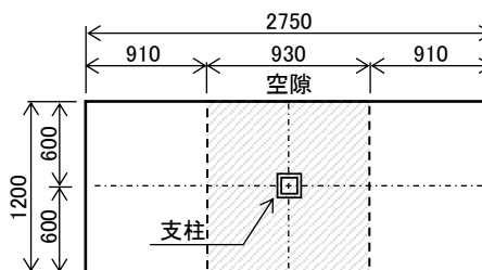
図-2 押し込み試験試験体
