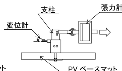
図-6 水平載荷試験
