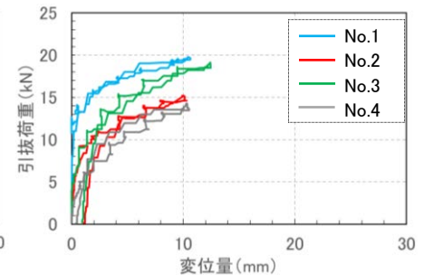
図-8 引張荷重と変位量(100 mm)
