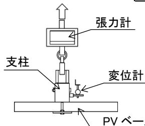
図-5 引張試験
