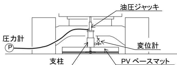
図-4 押し込み試験
