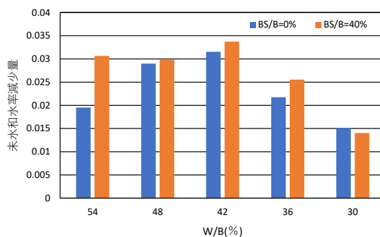
図-3 7-56 日の未水和水率の減少量
