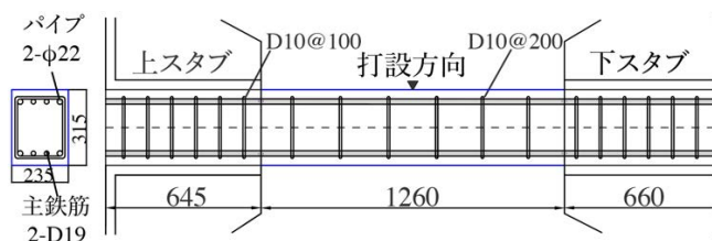
図1 試験体配筋図
