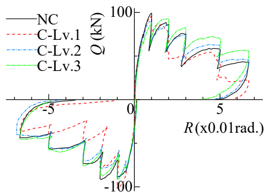
図3 包絡線
