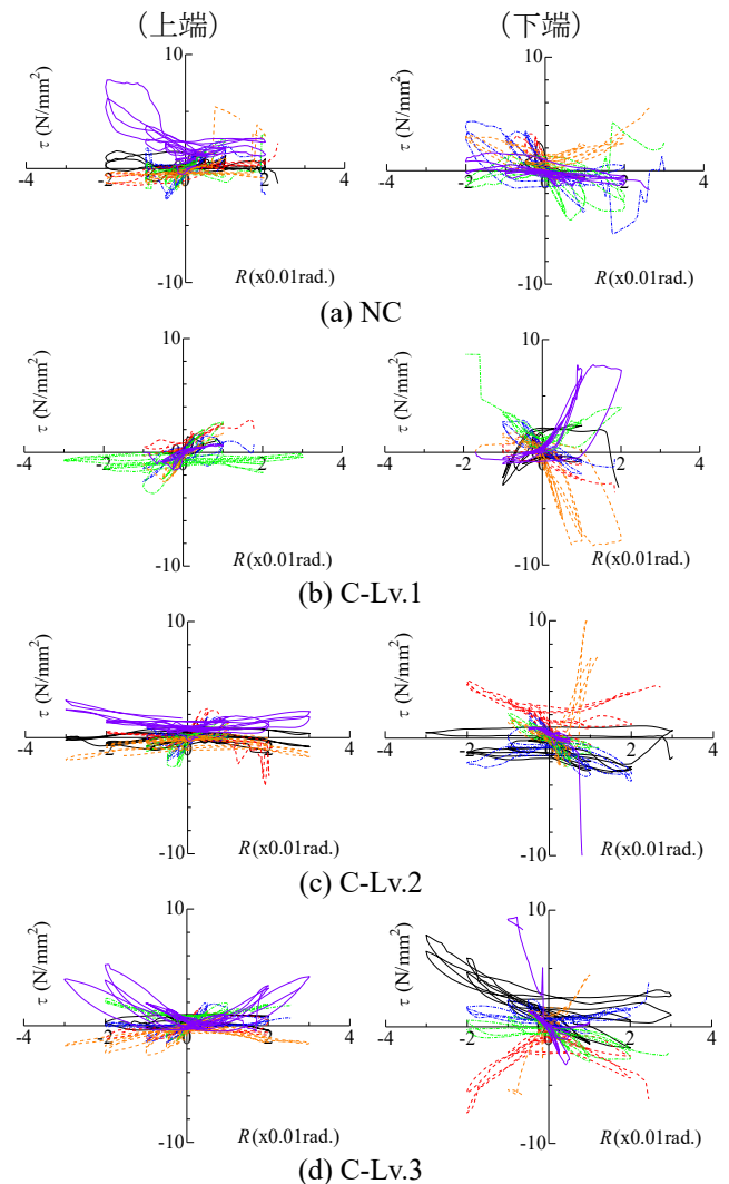
図 5 各試験体主鉄筋の付着応力-部材角関係
