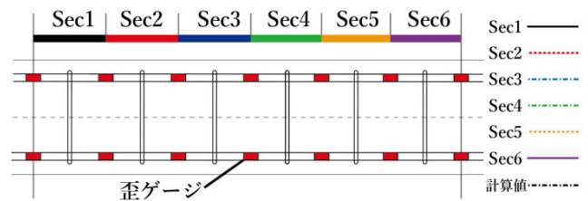
図 4 歪ゲージ貼付け位置と区間番号
