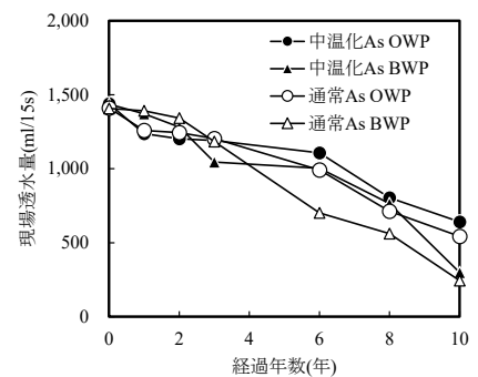
図6 透水量
