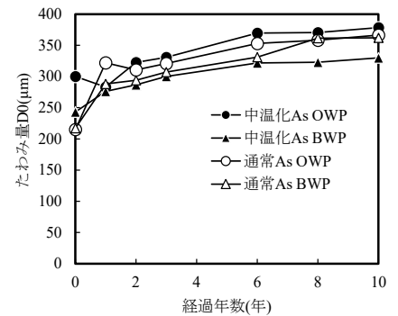
図4 たわみ量
