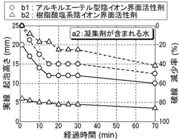
図-3 アルカリ溶液 a2:凝集剤が含まれる水での起泡性
