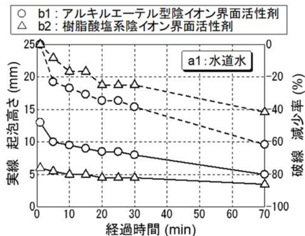
図-2 アルカリ溶液 a1:水道水での起泡性
