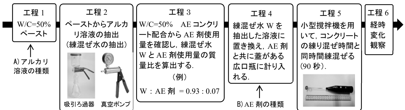
図-1 AE 剤の起泡性確認試験フロー
