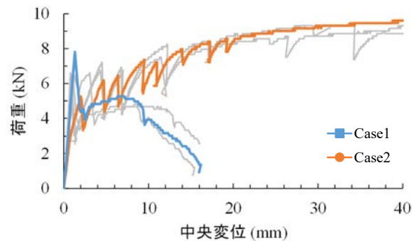
図-2 荷重—中央たわみ変位関係
