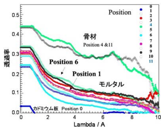
図-3 乾燥状態【重水】コンクリートの結果
