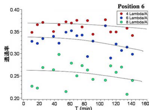
図-5 給水状態【重水】コンクリートの結果
