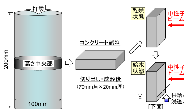
図-1 コンクリート試料の作製と測定時の設置概要
