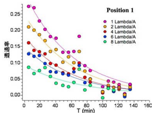
図-4 給水状態【重水】コンクリートの結果
