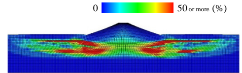
図7 せん断ひずみの解析結果 (無改良)
