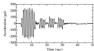
図2 入力地震波
