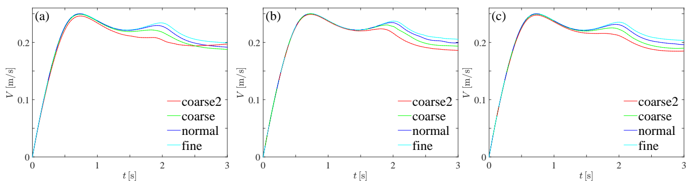
図 2: 2 次元気泡の上昇速度の経時変化: (a) ACLS, (b) CICSAM, (c) THINC/WLIC.
