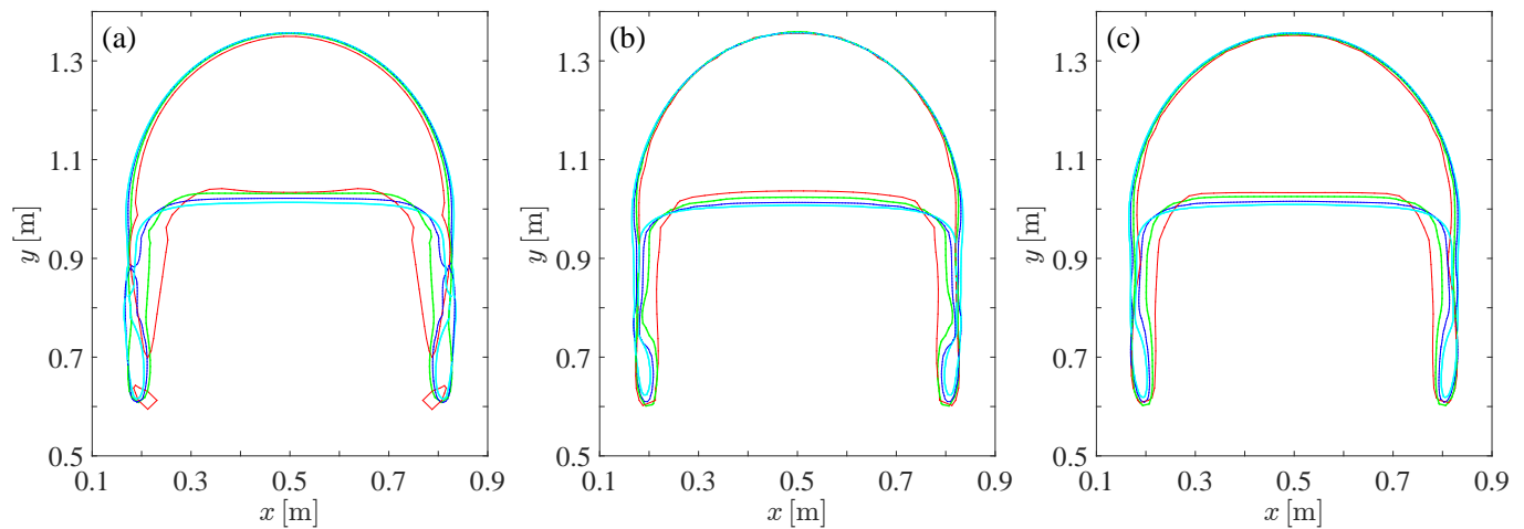
図 1: t = 3\text{s} における 2 次元気泡の形状: (a) ACLS, (b) CICSAM, (c) THINC/WLIC. 赤 - coarse2; 緑 - coarse; 青 - normal; シアン - fine.
