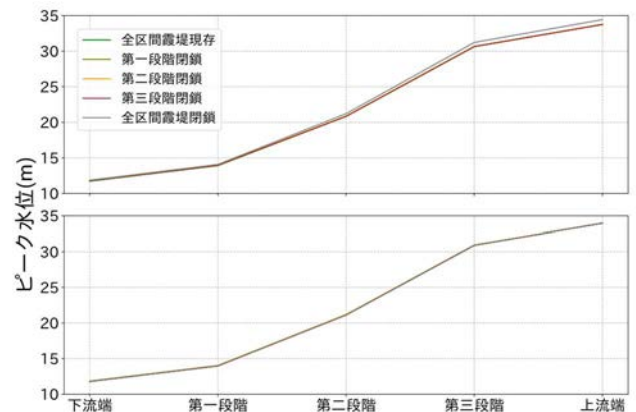
図-2 段階的の整備区間におけるピーク水位
