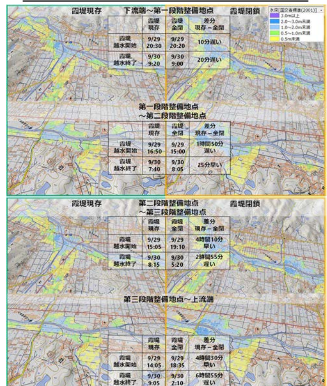
図-3 最大浸水深図と越水開始/終了時間
