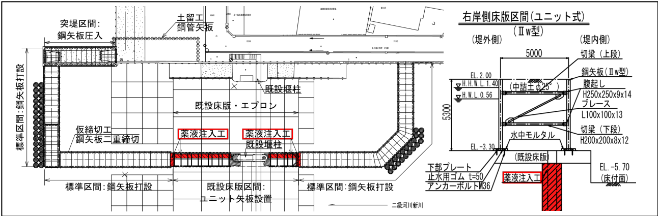
図－1 本工事における仮締切工の概要（右岸側施工時）
