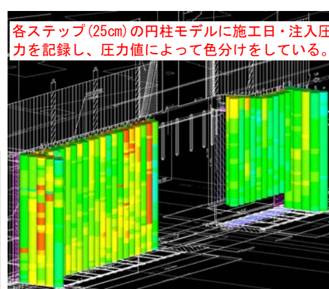
図-3 注入圧力のC I Mモデル
