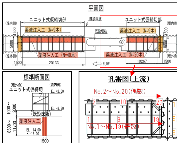
図-2 薬液注入工孔配置と標準断面図
