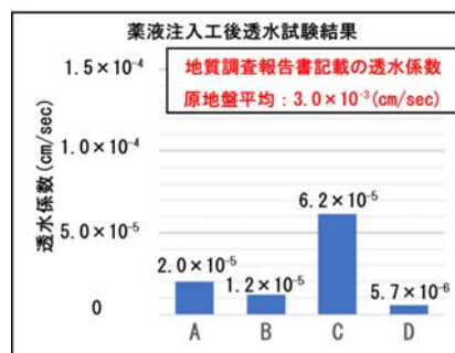
図-5 注入効果懸念箇所の現場透水試験結果
