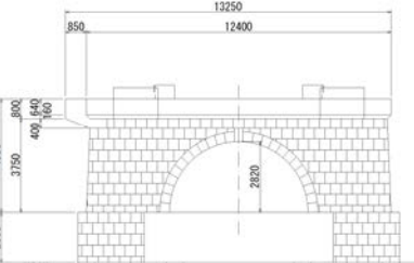
図-1 橋脚構造図
