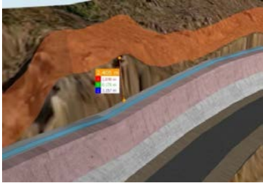
図-3 切土補強土壁の現況地盤との不整合箇所
