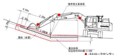
図2 掘削断面
