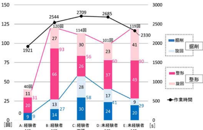
図 5 10m 当たりの作業回数・時間
