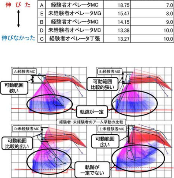
図 4 アーム挙動の比較
