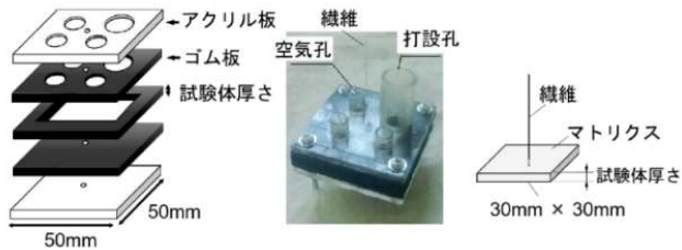
図－2 試験体および型枠形状
