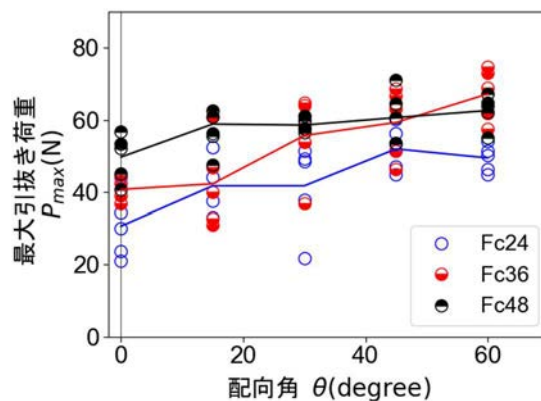
図-6 最大引抜き荷重と繊維配向角
