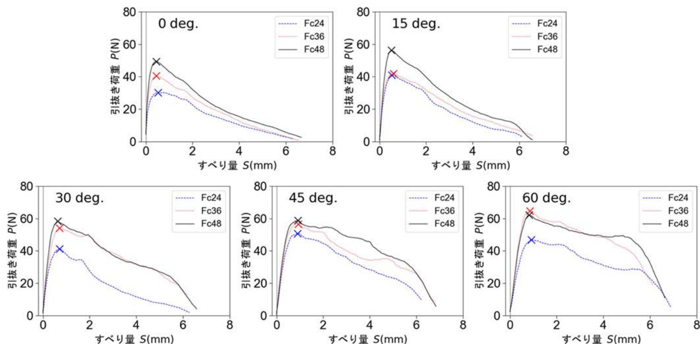
図-5 引抜き試験結果 (×:最大引抜き荷重)
