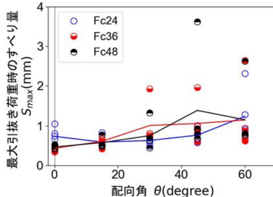
図-7 最大引抜き荷重時のすべり量と繊維配向角
