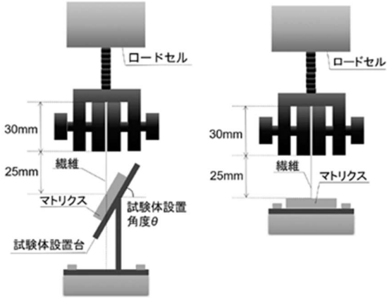
図－3 加力方法
