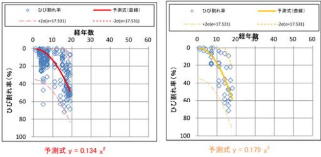
図-1 全体の劣化曲線(例) 図-2 一般の劣化曲線(例)
