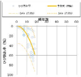
図-4 全体の劣化曲線(例)
