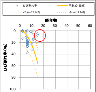
図-6 古い箇所で損傷が少ない例
