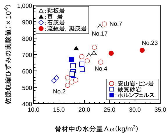
図2 骨材中の水分量と乾燥収縮ひずみの関係
