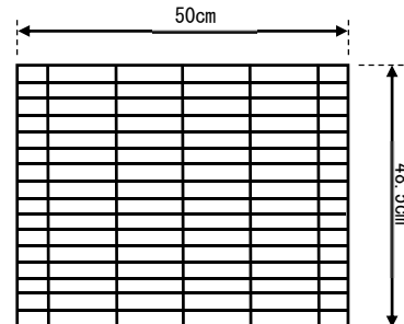
図2 シミュレーションに用いた雨水樹のC3タイプ雨水樹蓋（鋼製）
