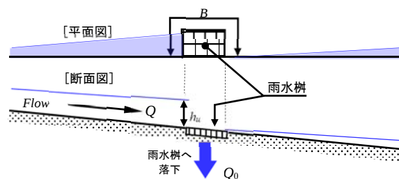
図 3 雨水樹への落下に関する記号の定義
