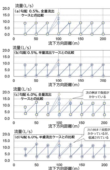
図 6 流量の流下方向への変化 (凡例は図 5 と同一)
