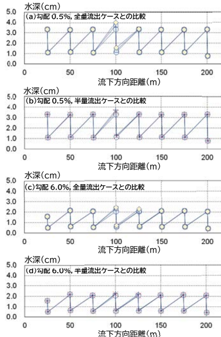
図 5 水深の流下方向への変化
