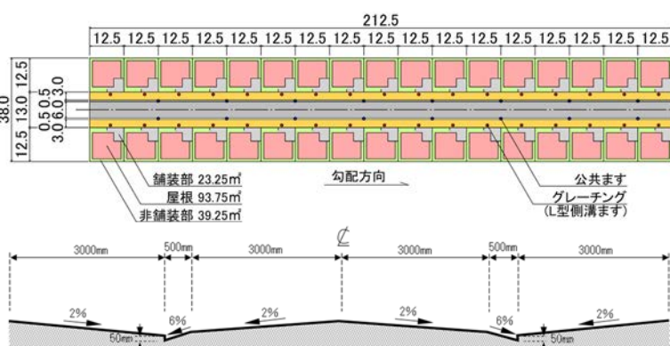
図1 数値シミュレーションで用いたモデル住宅地と街路（上：平面図、下：断面図）
