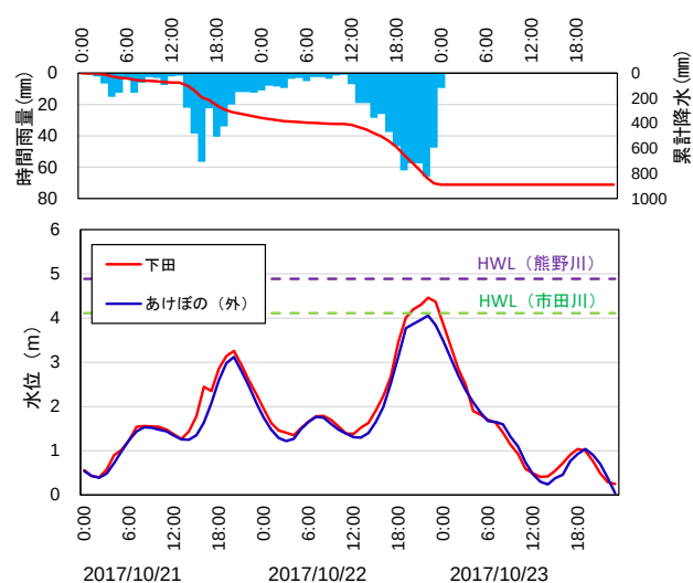
図 1 雨量と観測所水位
