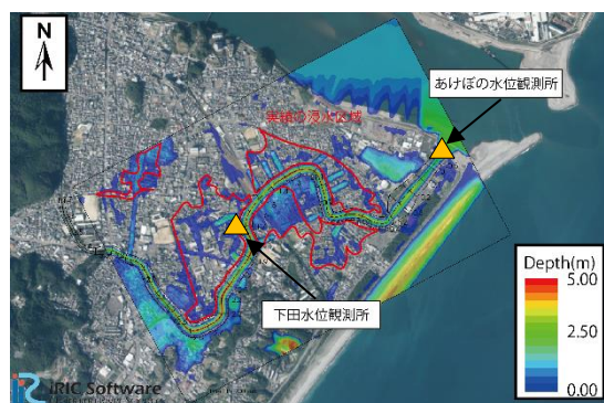
図 2 浸水範囲の計算結果と実績範囲のとの比較 （下流端水位条件：上側が実績、下側が天文潮位）
