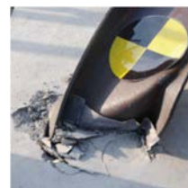
(c) PS 試験体基部
