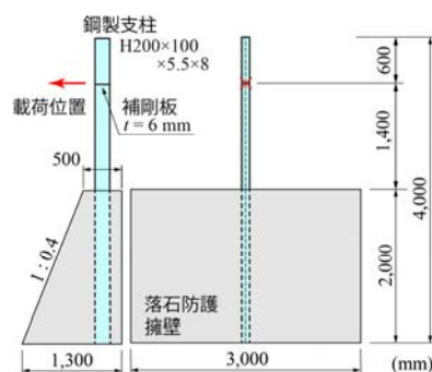
図-1 形状寸法
