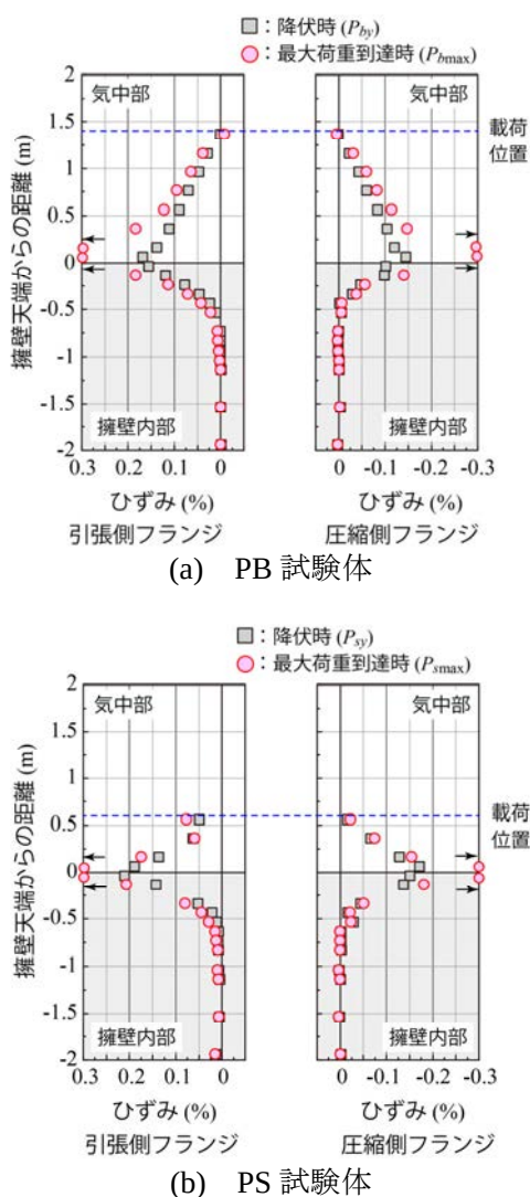
図-3 各時点における支柱縁ひずみ分布
