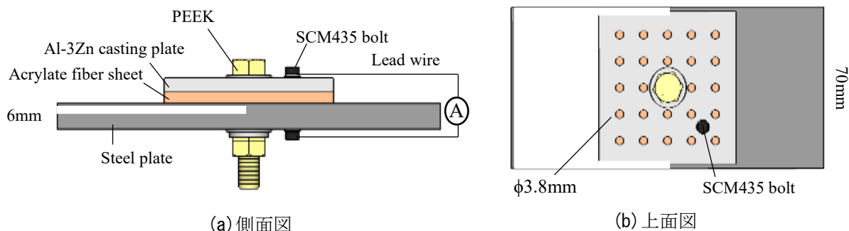
図-2 モデル試験体の概略図
