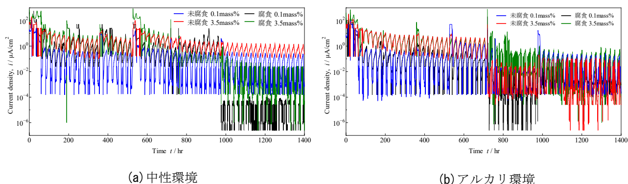
図-3 中性とアルカリ環境における電流密度の経時変化
