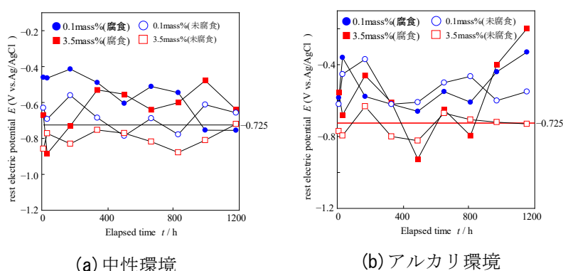
図-4 中性とアルカリ環境における電位の経時変化
