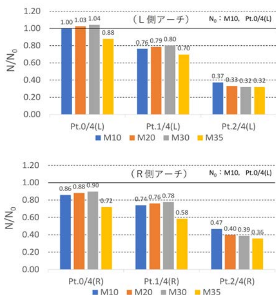
図-5 アーチ軸力 (地震時)
