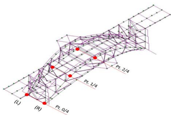
図-4 軸力図 (M35, 地震時)
