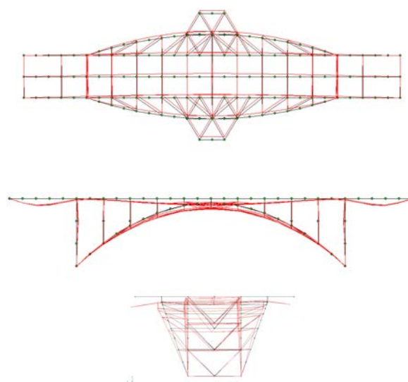
図-6 変形図 (地震時, モデル M35)
